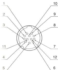
KS101-15/KS101-20/KS101-20MS
