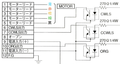
KS101-15/KS101-20/KS101-20MS
